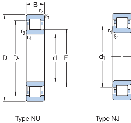
Type NU
