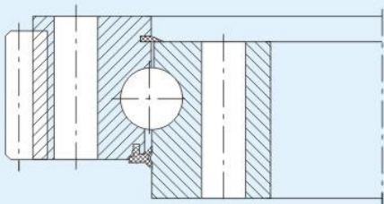
外齿式 With outer gear
